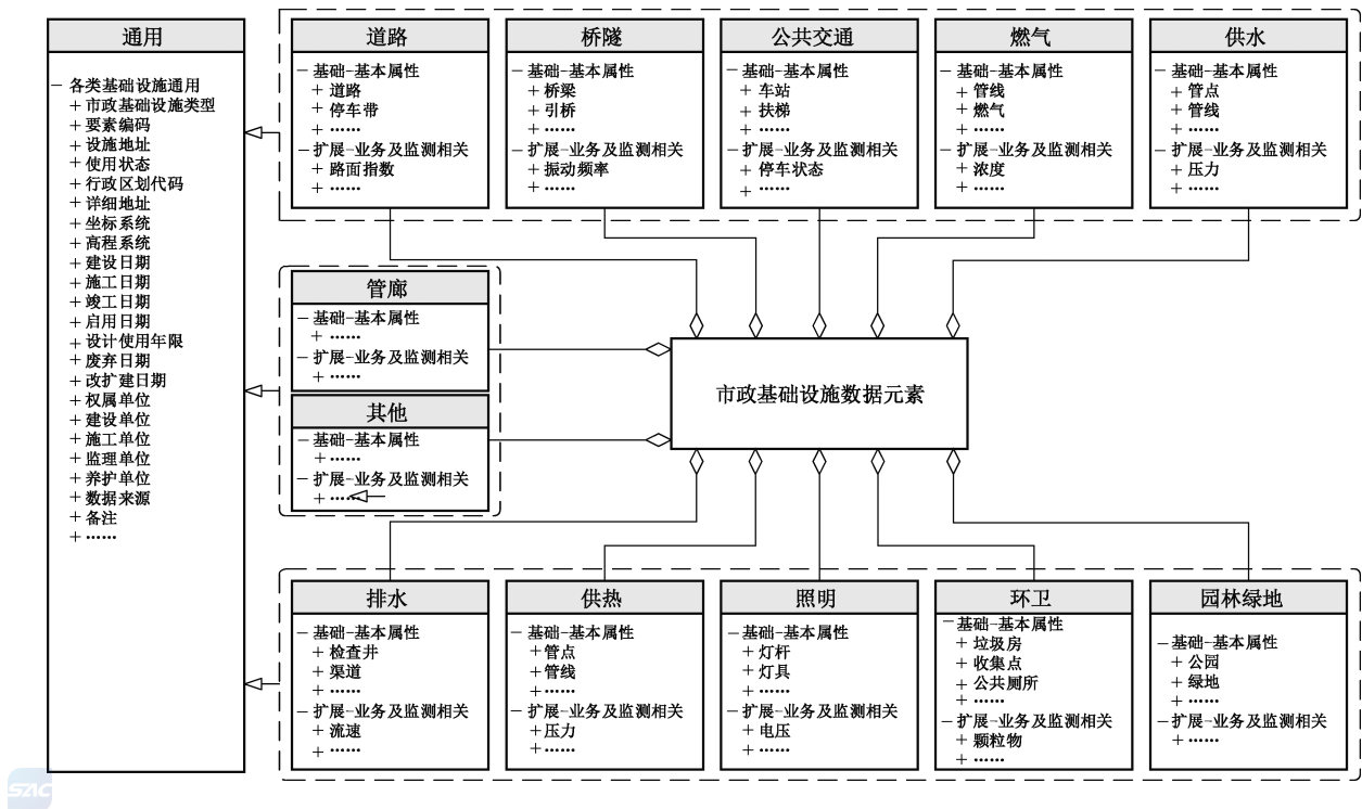
图 1 市政基础设施数据元素逻辑模型
